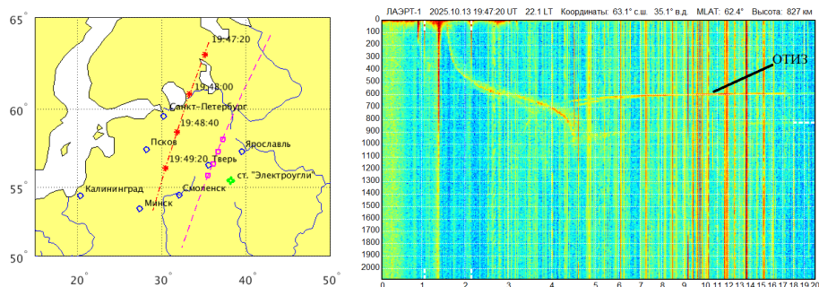
Рисунок 1 – слева карта с демонстрацией следов орбиты КА «Ионосфера-М», справа – ионограмма ионозонда ЛАЗЭРТ-1 со следом ОТИЗ.
