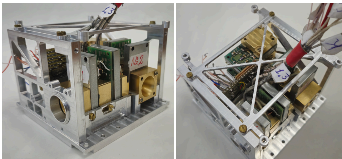
Рис. 1а, б. Фотографии детекторной системы КОДИЗ-2 в сборке спутника.
