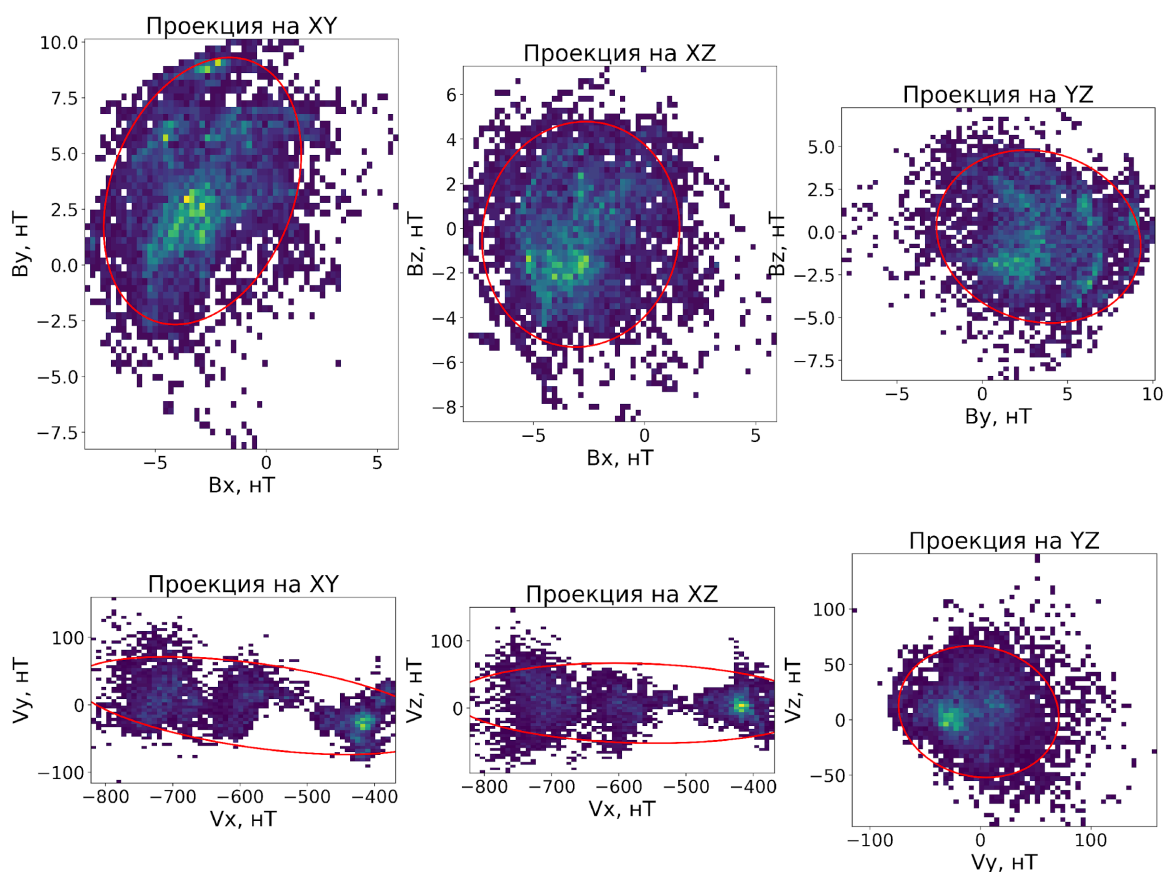
Рис .1 Примеры проекционных отображений для двух векторных полей \mathbf{V} и \mathbf{B} .
