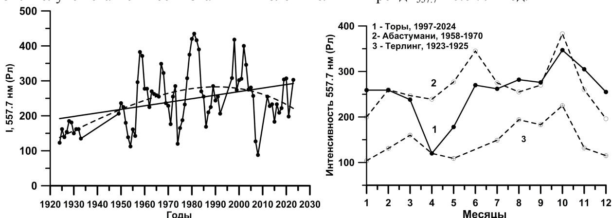
Рис.1 Многолетние вариации среднегодовых значений I_{557.7} (слева) и сезонные ходы в различные периоды наблюдений в 20-21 веках на 3-х среднеширотных станциях (справа).
