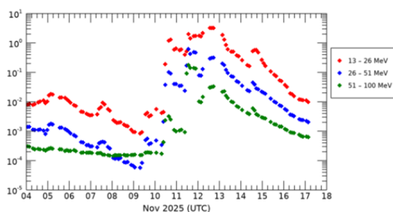
Рис.1.Хронология потока протонов в точкеL1. потока лёгких ядер в точке L1. по данным ERNE Sensor Unit (ESU)
