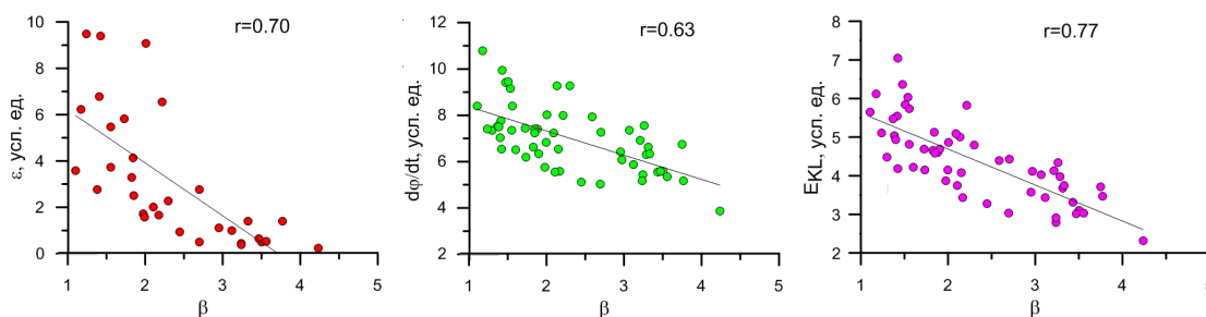
Рис. 1. Зависимости \epsilon , d\phi/dt и E_{KL} от параметра \beta (среднегодовые значения). r – коэффициенты линейной корреляции.
