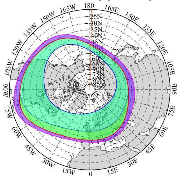
Dst = -590, AL = -1800 Дата 1989.03.14, UT = 00:15 Зоны ОПС и высыпаний. Географические координаты
