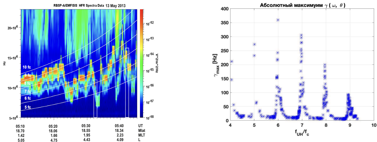
Рис. 1. Часть спектрограммы, отображающая временной интервал 05:10–05:45 UT (слева). Максимальный инкремент нарастания ВГР волн вдоль орбиты спутника, параметризованный величиной f_{UH}/f_c (справа).
