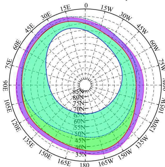
Dst = -590, AL = -1800 Зоны ОПС и высыпаний. CGM-координаты
