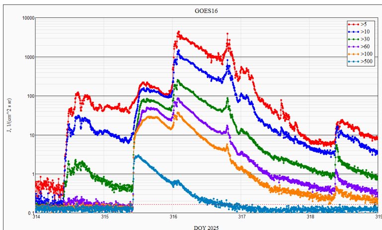
Рис. 1 Временные профили потоков солнечных протонов по данным ИСЗ GOES 10-14.11.2025
