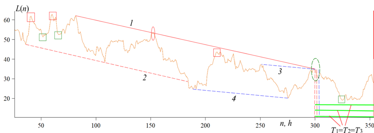
Рис. 1. Зависимость L(n) характеризует уровень хаоса для интенсивности измерений рентгеновского излучения Солнца. Красная вертикальная прямая линия отвечает моменту вспышки класса X1.8, которая имела место 4 ноября 2025 года.
