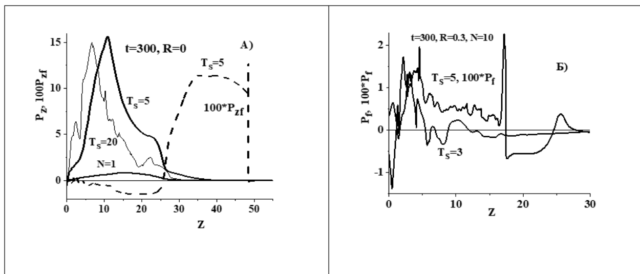
А) Продольный импульс струи ( P_Z ) и МКВ ( P_{Zf} ) на оси симметрии в момент времени t = 300 N = 1 и N = 10 . Б) Азимутальный импульс струи. Критерии не выполняются для T_s = 5 .
