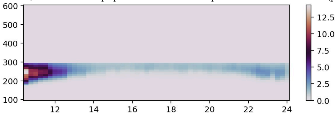
Рисунок 1. Высотный профиль ночного хода интенсивности линии 630 нм за счет диссоциативной рекомбинации O_2^+ . Взяты среднесезонные значения осени 2022 года.
