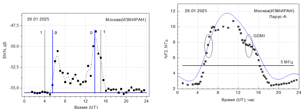
Рис. 1. Зависимость фонового ЭМ шума в зимний сезон (26.01.2025): эксперимент (левая панель) и состояние ионосферы – foF2 на ст. ИЗМИРАН (правая панель, модель GDM – сплошная линия, квадратиками нанесены данные ионозонда “Парус-А”, и горизонтальная линия соответствует частоте 5 МГц). Вертикальными линиями отмечены времена прохождения утреннего и вечернего терминаторов (0 и 100 км высоты).
