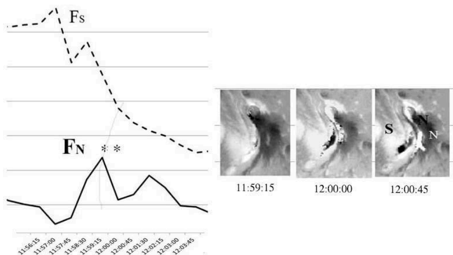
Рис. 1. Звездочками отмечен интервал времени, в котором произошло синхронное уменьшение магнитного потока обеих полярностей, соответствующее гашению потока.
